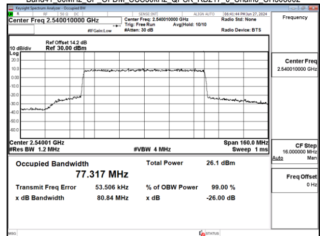
Band41 80MHz CP OFDM_SCS30kHz QPSK_RB217_0 Chain0_CH508002
