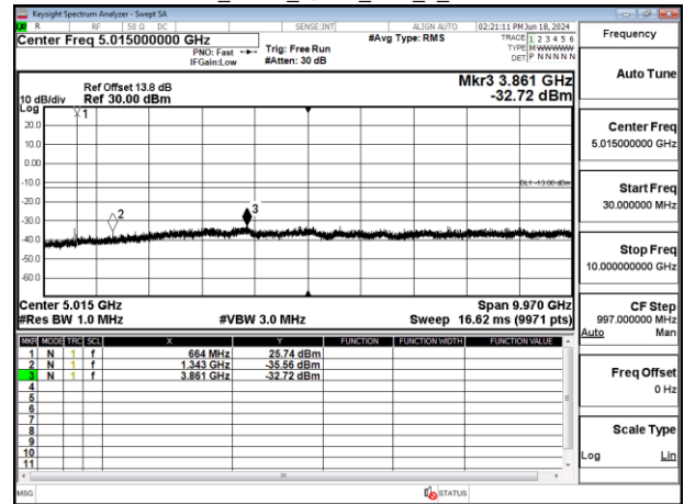
Band71_5MHz_QPSK_RB1_0_CH133297
