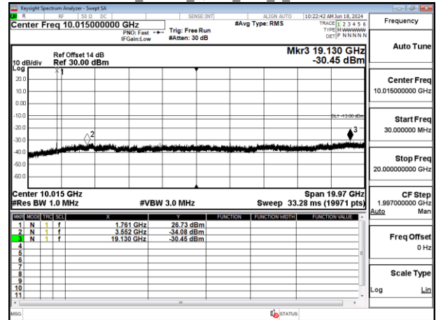
Band71_5MHz_QPSK_RB1_0_CH133147
