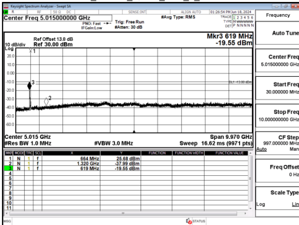
Band71_20MHz_QPSK_RB1_0_CH133297
