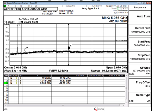
Band71_5MHz_QPSK_RB1_0_CH133297
