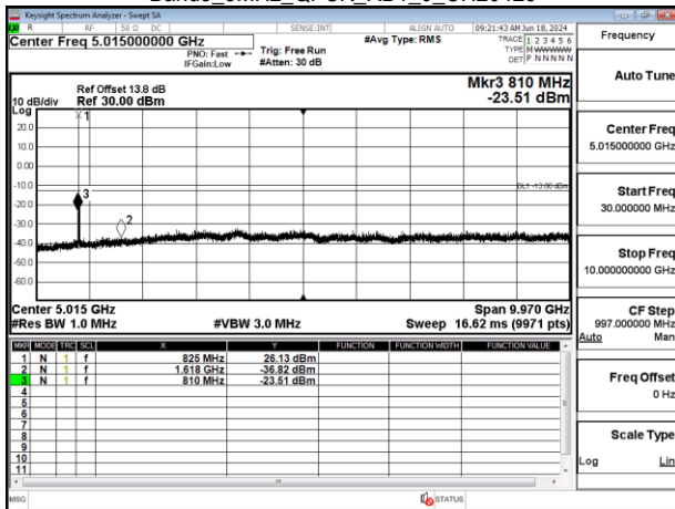
Band5_5MHz_QPSK_RB1_0_CH20525
