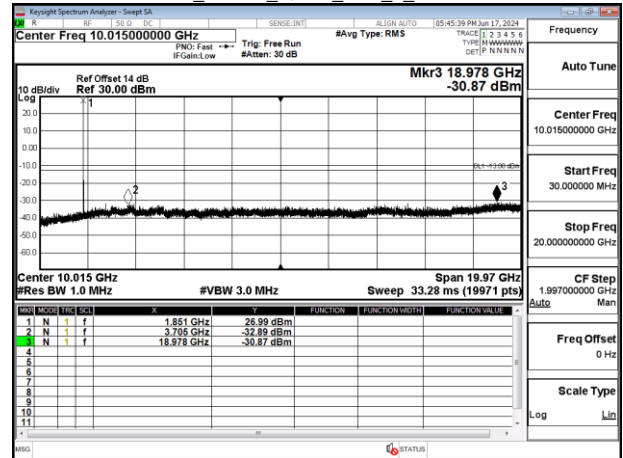
Band2_20MHz_QPSK_RB1_0_CH18900
