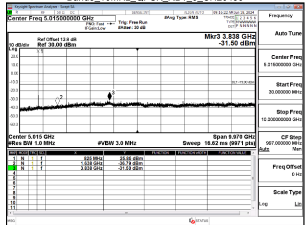
Band5_10MHz_QPSK_RB1_0_CH20525
