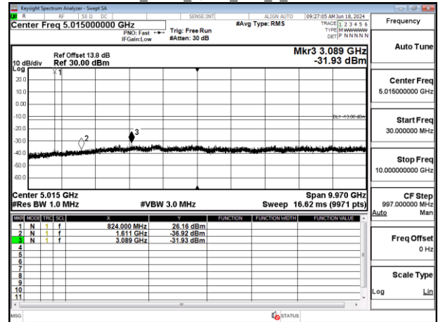
Band5_3MHz_QPSK_RB1_0_CH20525
