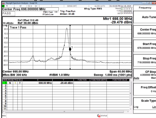
Band Edge_Band71_20MHz_QPSK_RB100_0_CH133222
