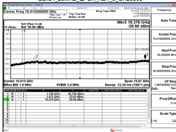
Band4_20MHz_QPSK_RB1_0_CH20300
