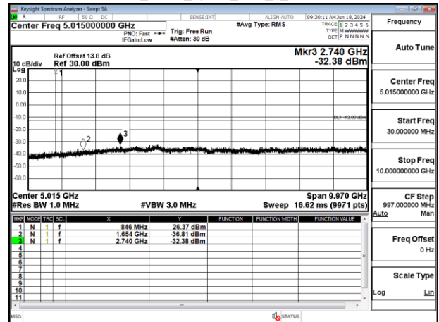
Band5_3MHz_QPSK_RB1_0_CH20635
