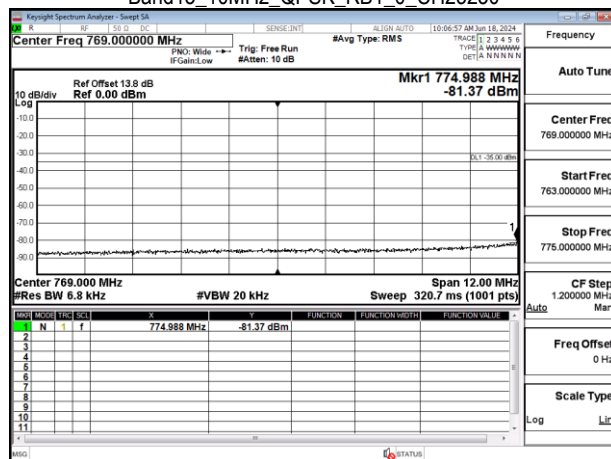
Band13_10MHz_QPSK_RB1_0_CH23230
