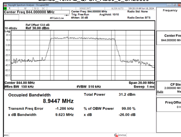
Band5_10MHz_QPSK_RB50_0_CH20600
