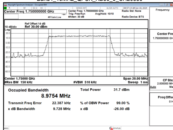
Band4_10MHz_QPSK_RB50_0_CH20350
