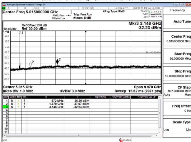
Band71_20MHz_QPSK_RB1_0_CH133297
