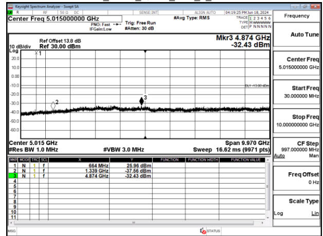
Band71_5MHz_QPSK_RB1_0_CH133297
