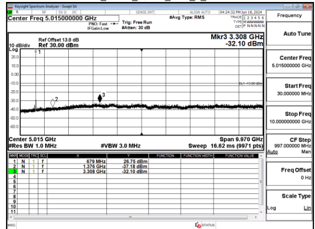
Band71_5MHz_QPSK_RB1_0_CH133297
