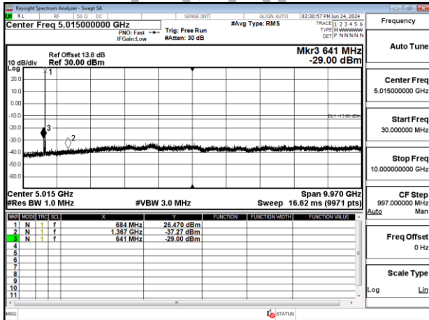
Band71_20MHz_QPSK_RB1_0_CH133222
