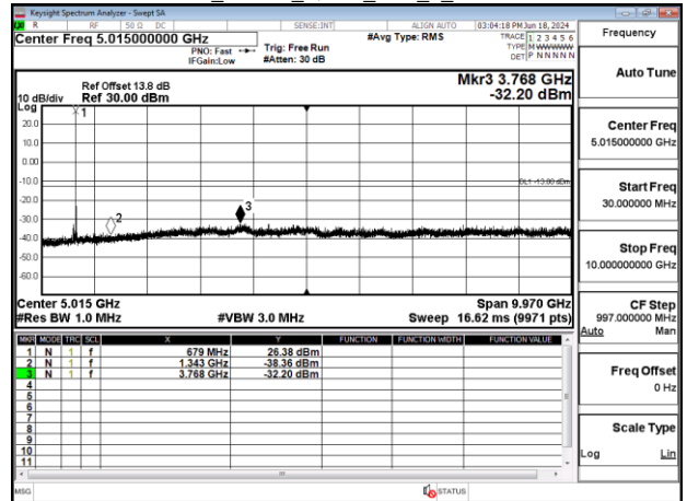
Band71_20MHz_QPSK_RB1_0_CH133372
