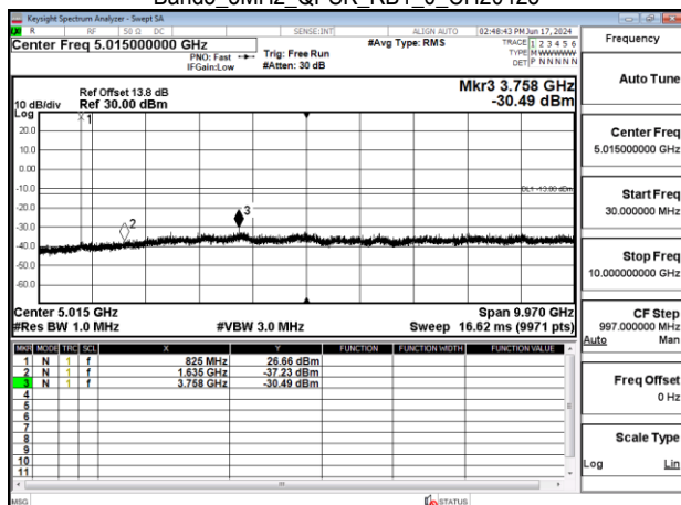
Band5_5MHz_QPSK_RB1_0_CH20525
