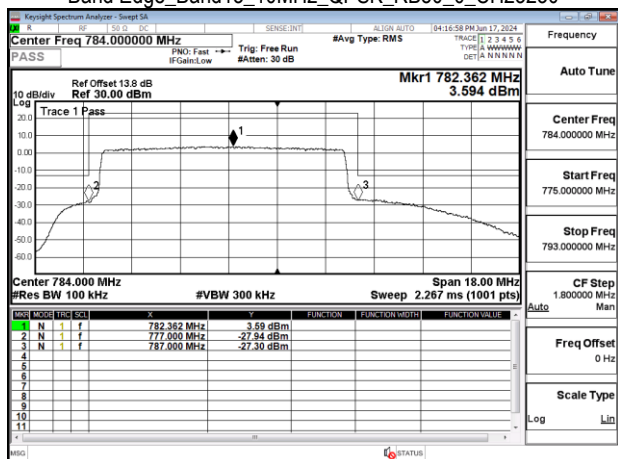
Band Edge_Band13_10MHz_QPSK_RB50_0_CH23230
