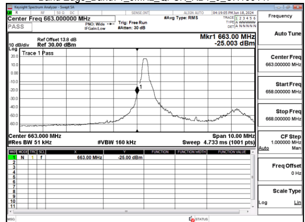
Band Edge_Band71_5MHz_QPSK_RB1_0_CH133147
