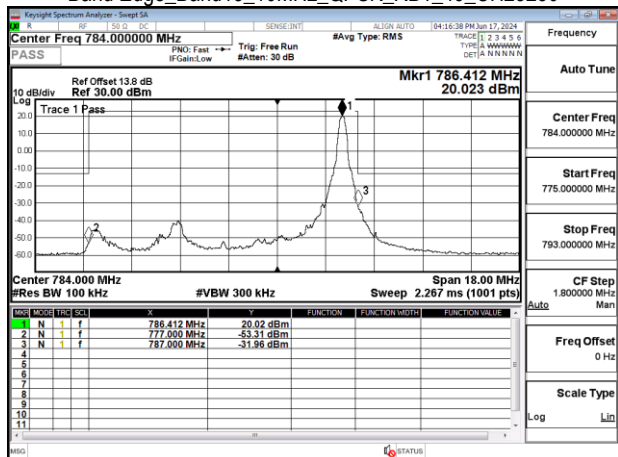
Band Edge_Band13_10MHz_QPSK_RB50_0_CH23230
