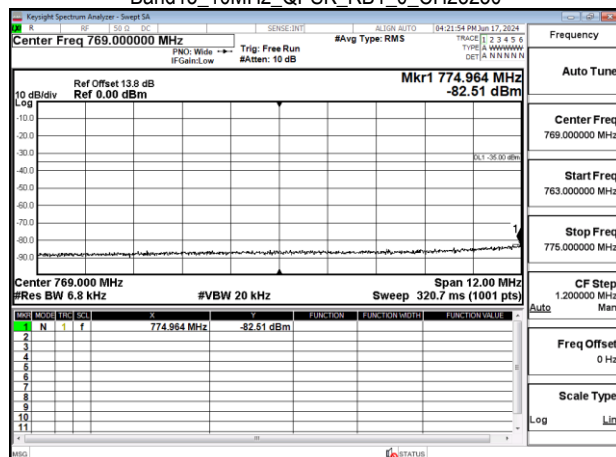
Band13_10MHz_QPSK_RB1_0_CH23230
