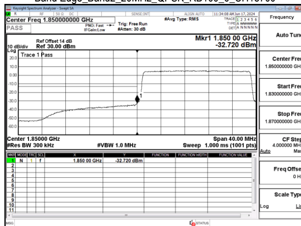
Band Edge_Band2_20MHz_QPSK_RB100_0_CH19100
