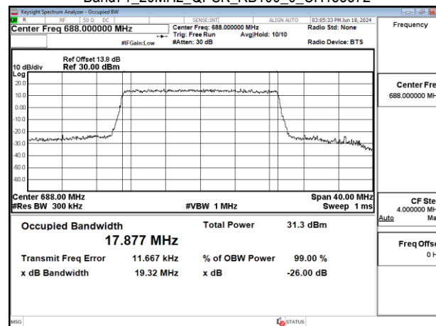
Band71_20MHz_QPSK_RB100_0_CH133372
