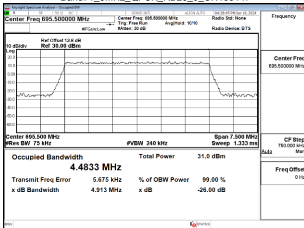
Band71_5MHz_QPSK_RB25_0_CH133447
