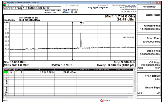
WCDMA_B4_LowCH1312-1712.4
