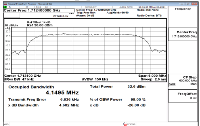
HSUPA_B4_LowCH1312-1712.4
