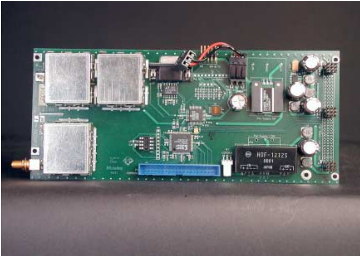
930-12693-01 IF Controller
