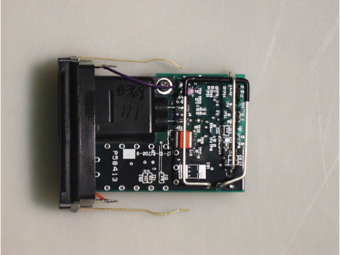
PCB BOTTOM
