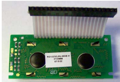
LCD Bottom
