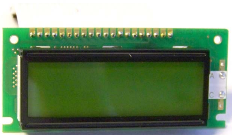
LCD Top
