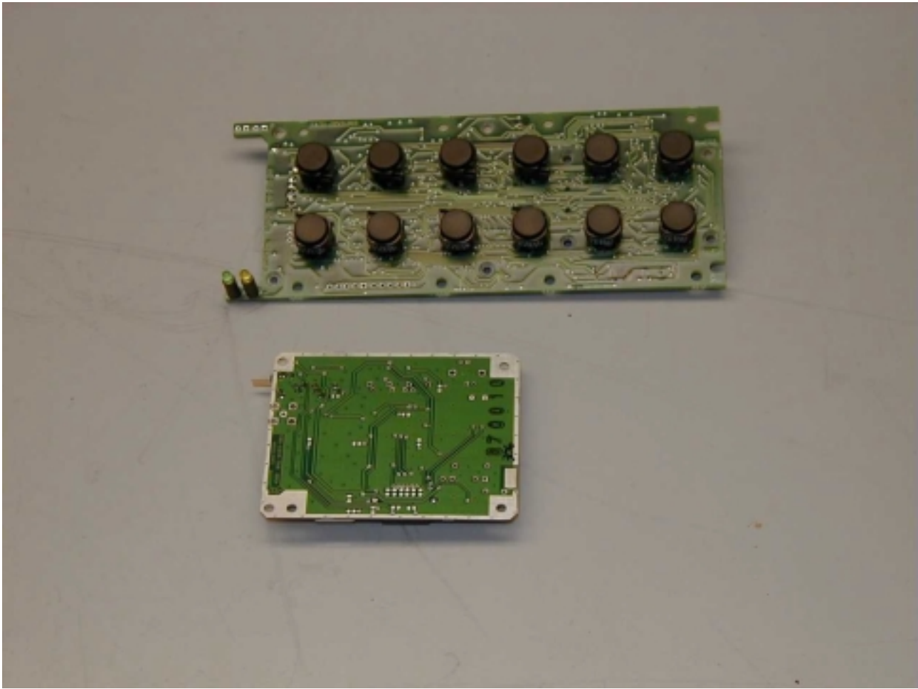
PCB Bottom
