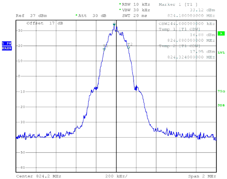
(Plot E2: EDGE 850MHz Channel = 128)
