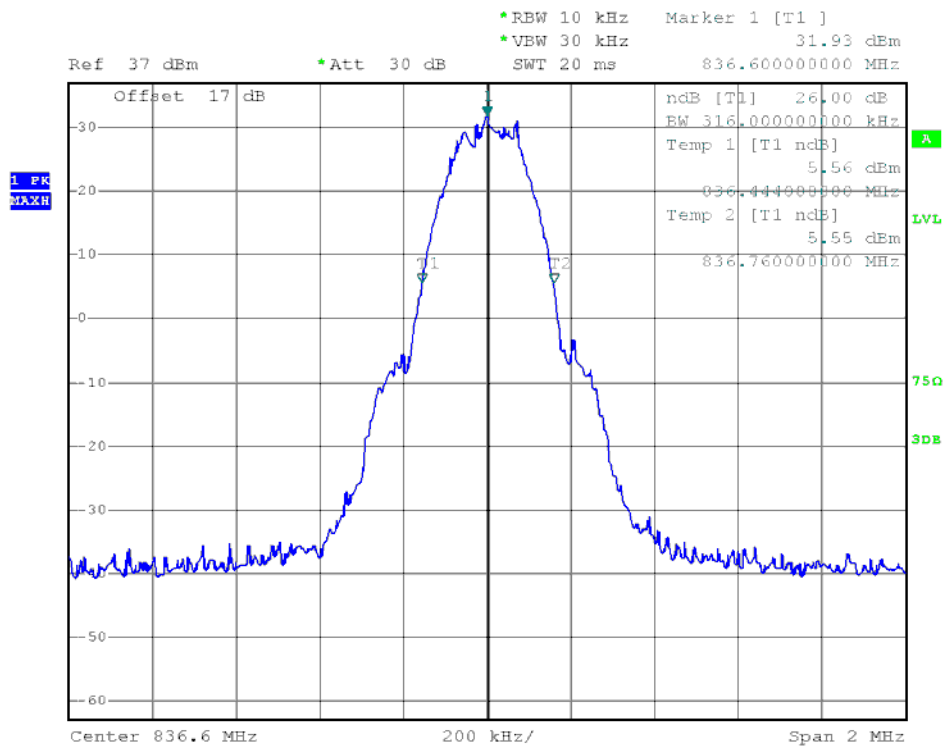
(Plot E3: EDGE 850MHz Channel = 190)
