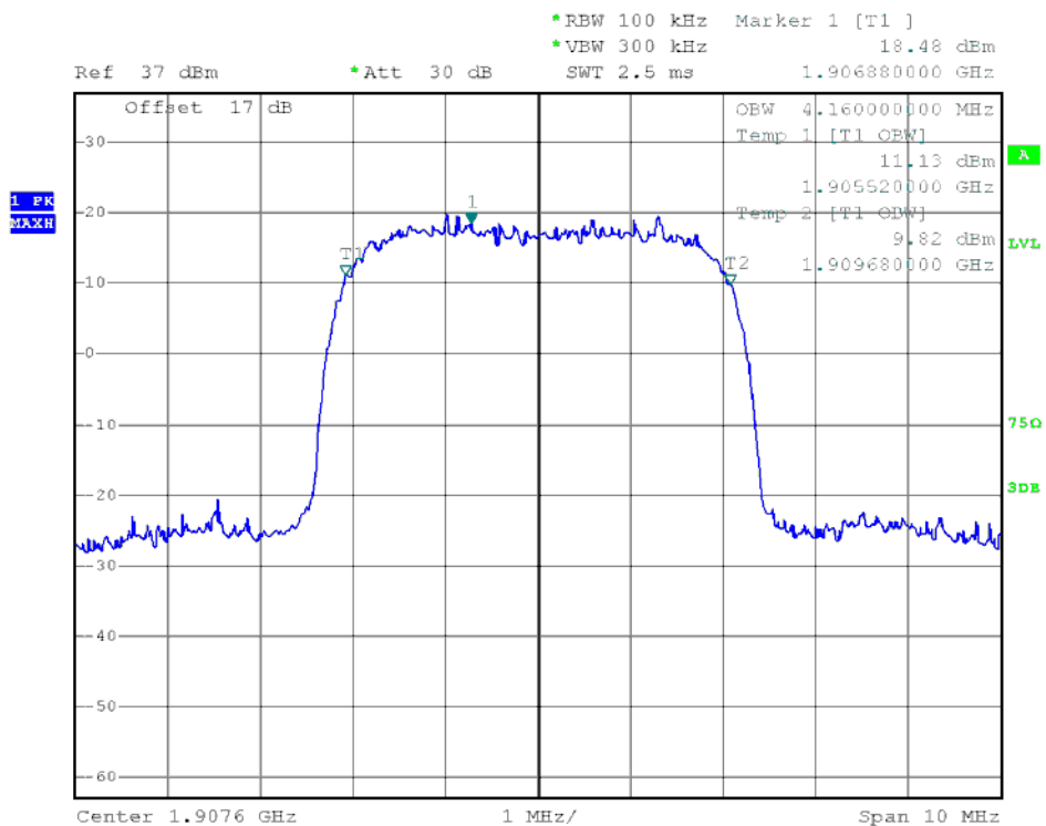
(Plot H6: WCDMA1900MHz Channel = 9538)
