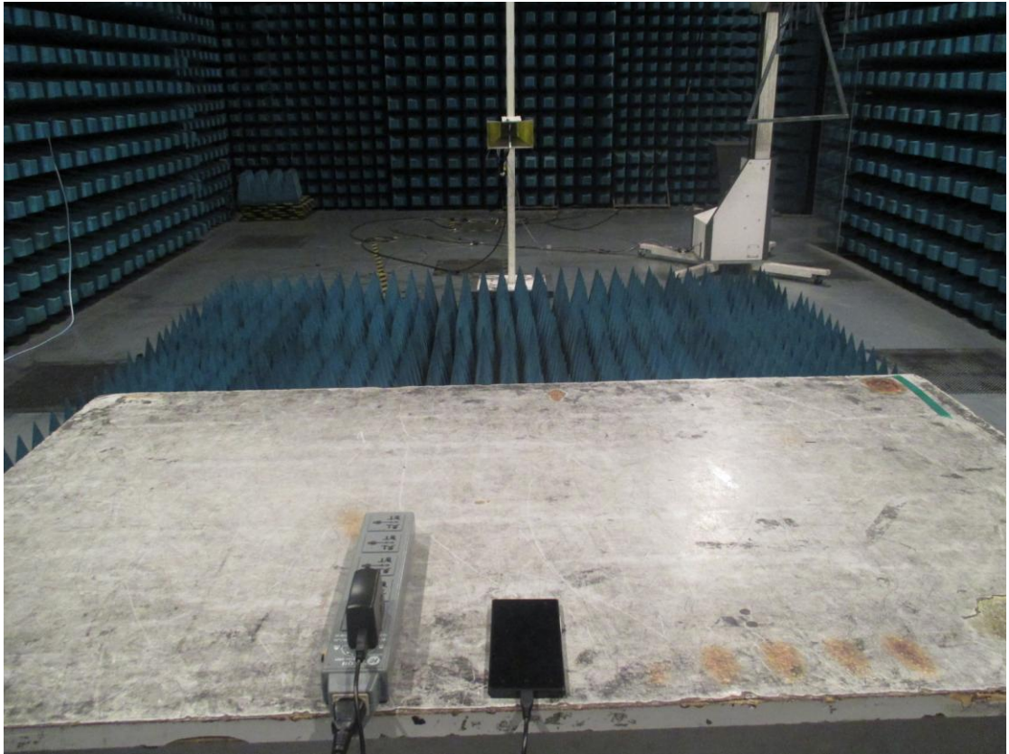
1GHz~18GHz
