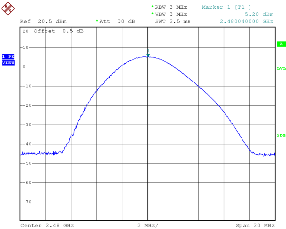
Plot B2: \pi/4 -DQPSK
