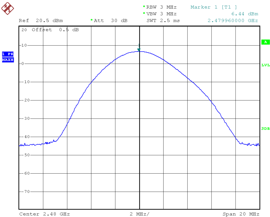
Plot B3: \pi/4 -DQPSK
