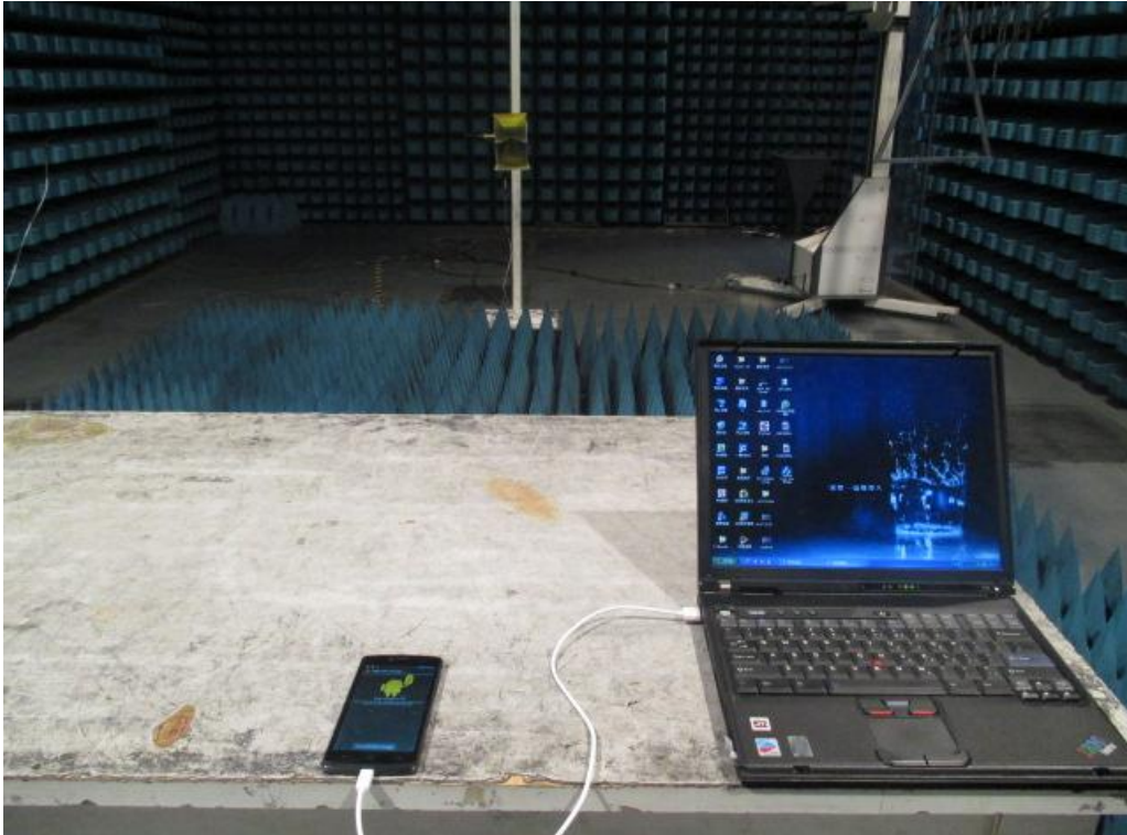
1GHz~18GHz
