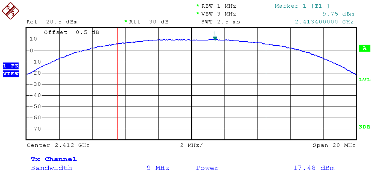
(Plot 2.2 A: Channel 1: 2412MHz @ 802.11b)
