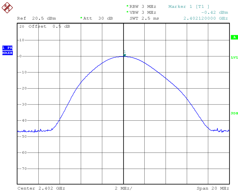
(Plot A: Channel 0: 2402MHz)
