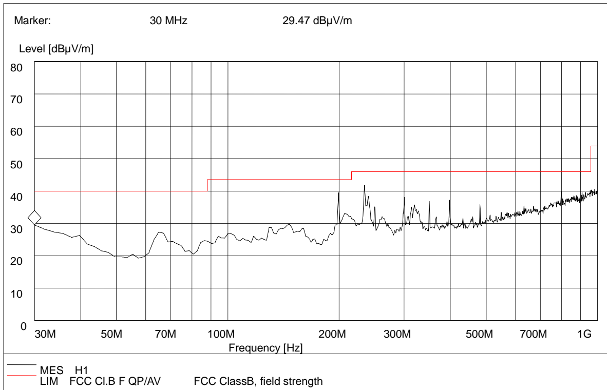
(Plot A: 30MHz to 1GHz, Antenna Horizontal)
