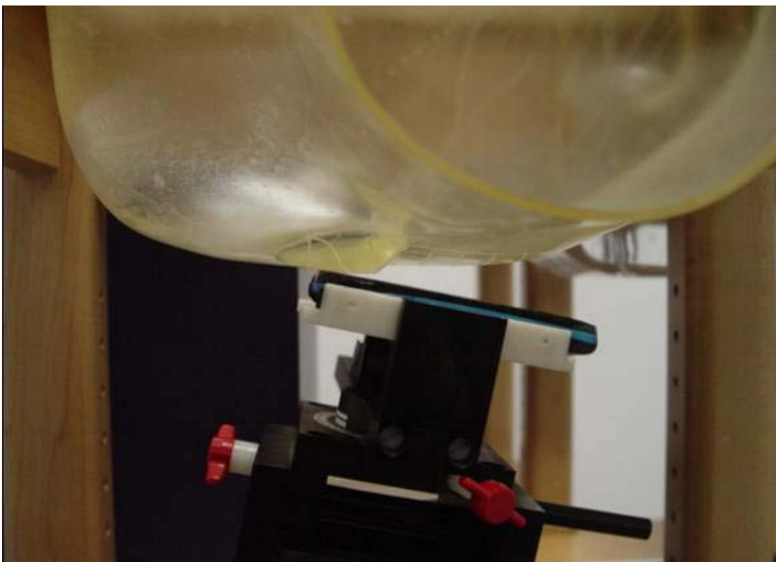
Left Head (EUT Tilt)
