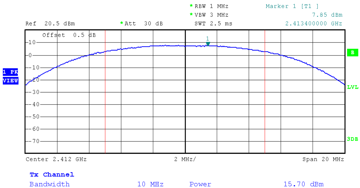
(Plot 2.2 A: Channel 1: 2412MHz @ 802.11b)
