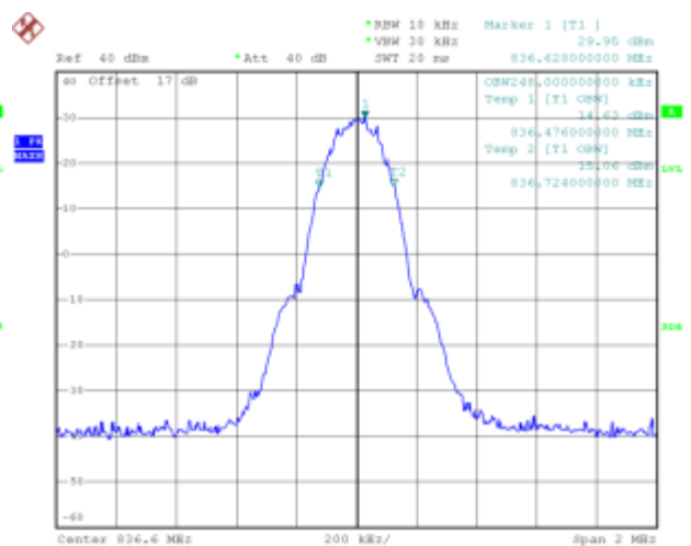
(Plot T: GSM 850MHz Channel = 190)
