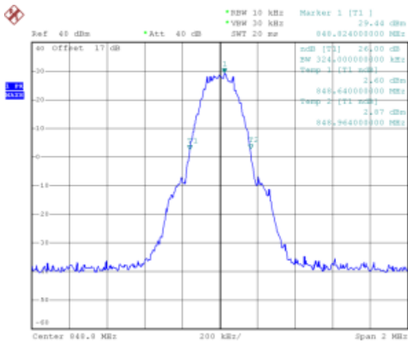
(Plot U: GSM 850MHz Channel = 251)
