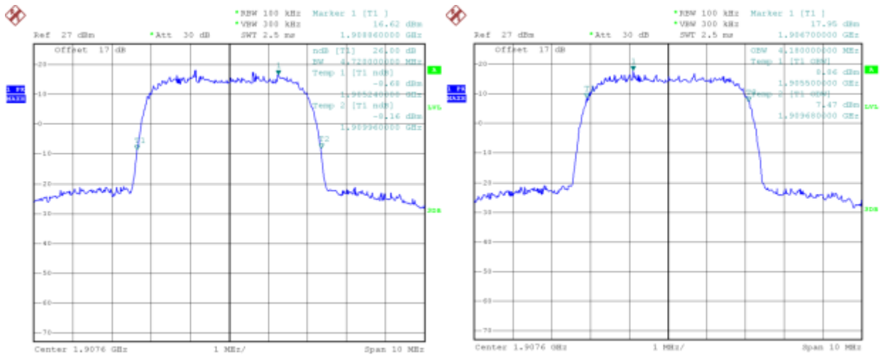
(Plot F: WCDMA1900MHz Channel = 9538)
