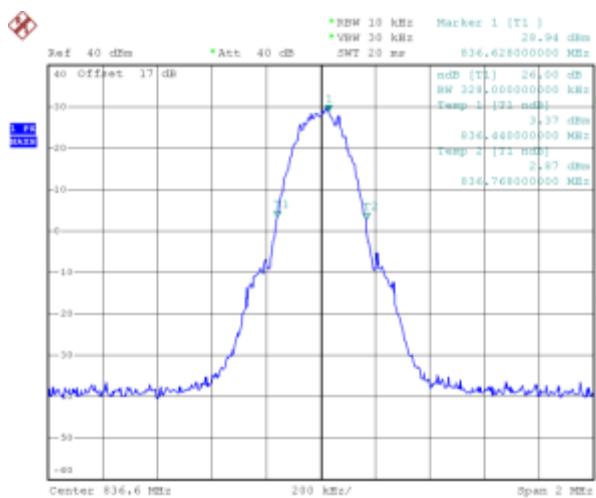
(Plot T: GSM 850MHz Channel = 190)
