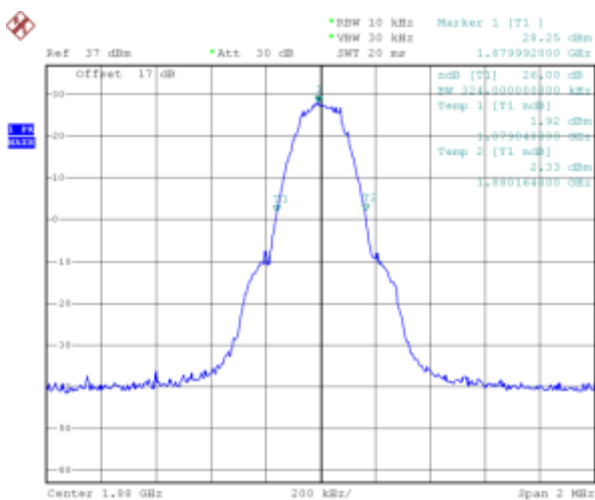
(Plot W: GSM 1900MHz Channel = 661)
