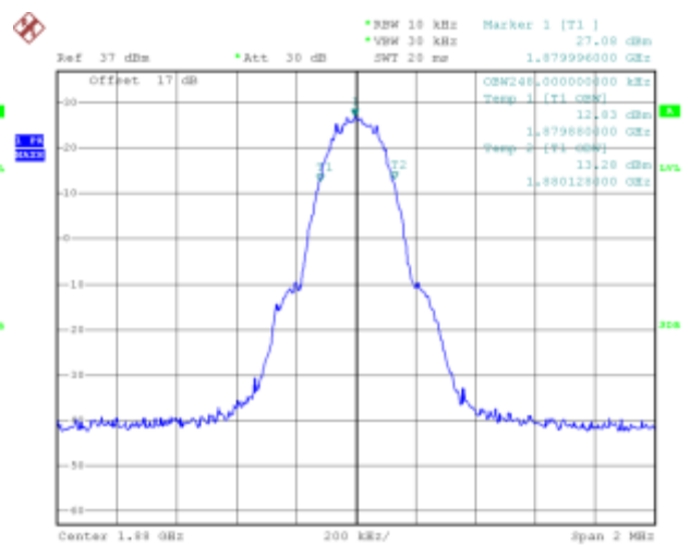
(Plot W: GSM 1900MHz Channel = 661)
