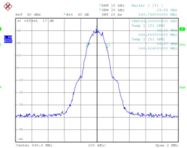
(Plot U: GSM 850MHz Channel = 251)
