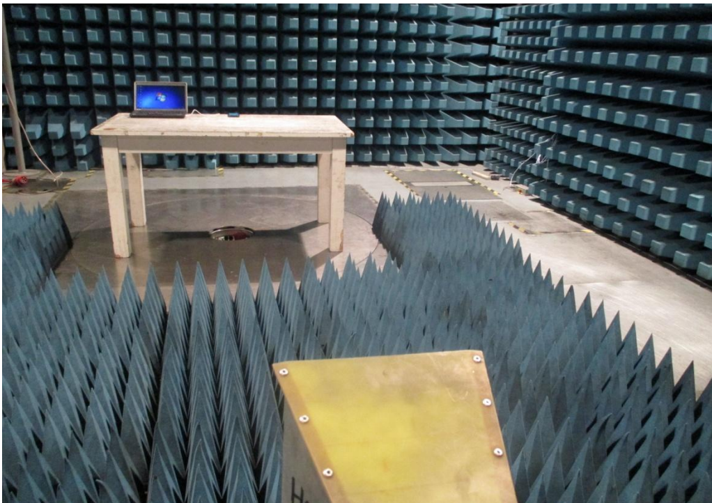
1GHz~18GHz
