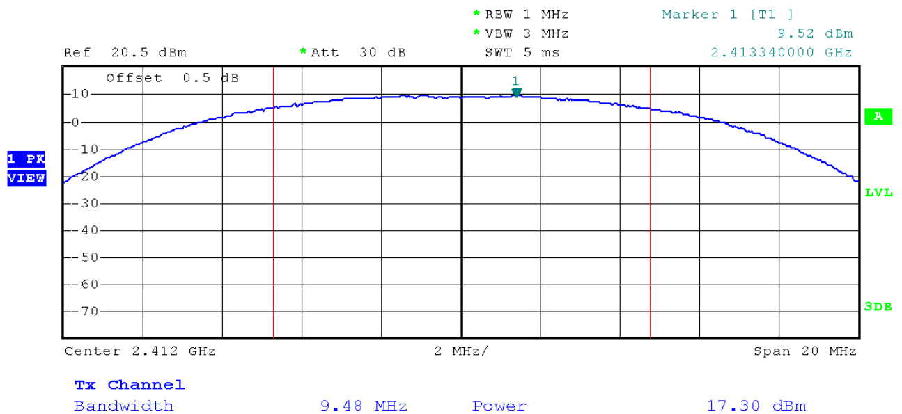
(Plot 2.2 A: Channel 1: 2412MHz @ 802.11b)
