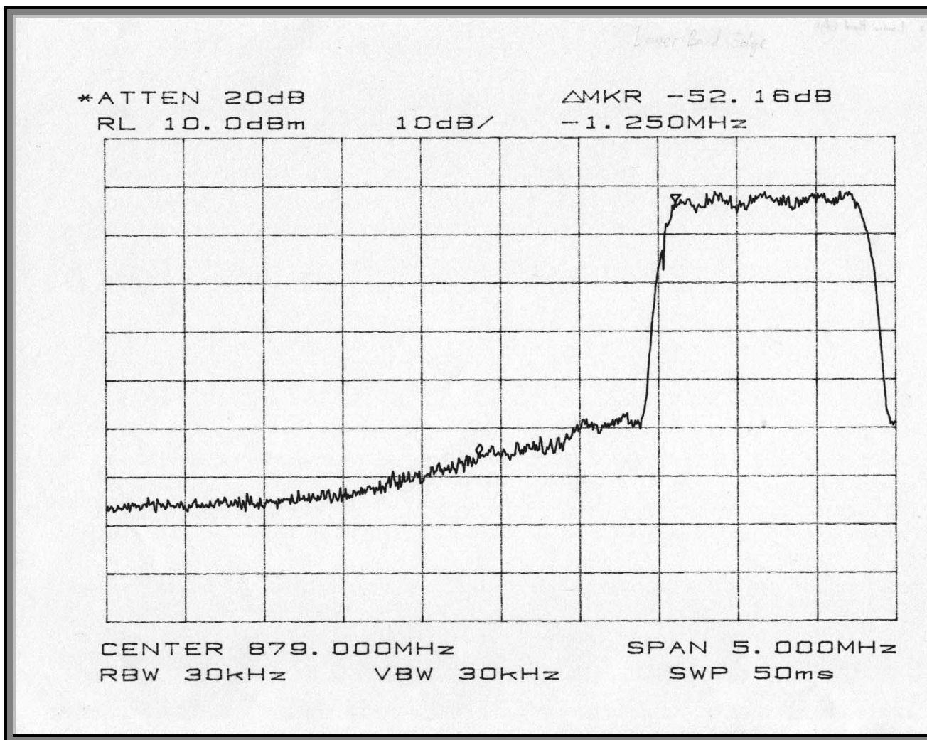
Lower Band Edge
