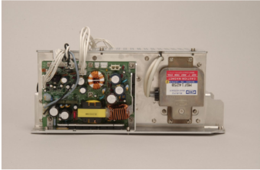
Magnetron Module
