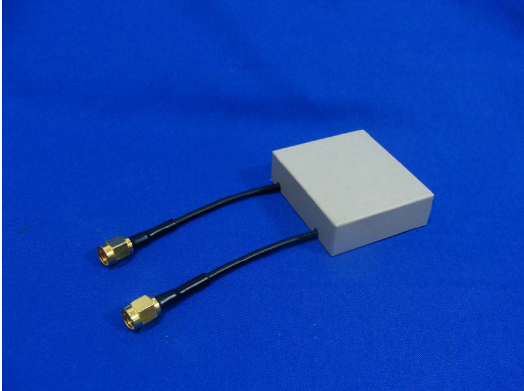
(12) EUT Photo - (Ant:IFA)
