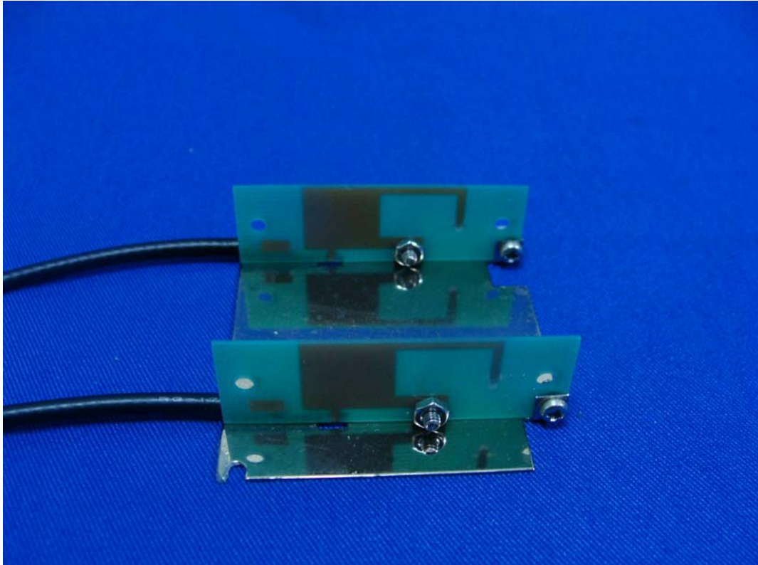
(16) EUT Photo - (Ant:IFA)
