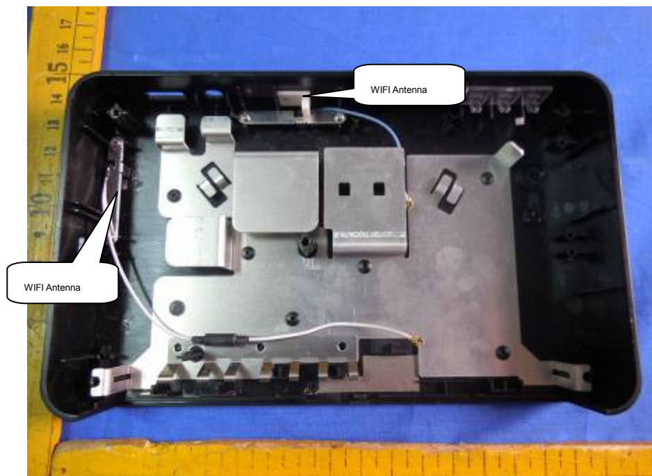
2) EUT Photo
