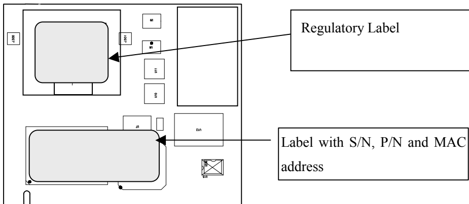
Mini PCI Label Placement (front side)
