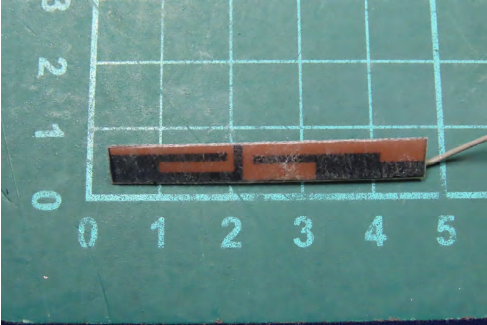
(36) EUT Photo
