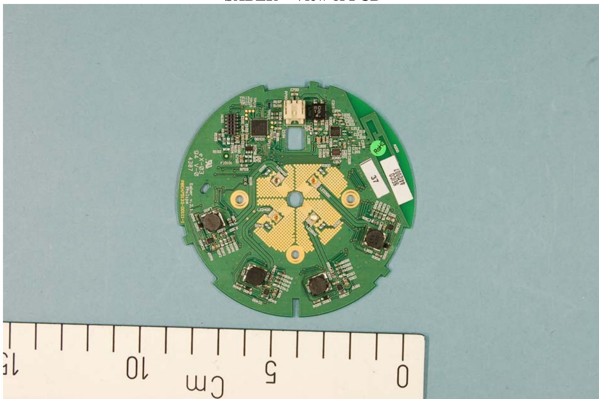
SABER – PCB
