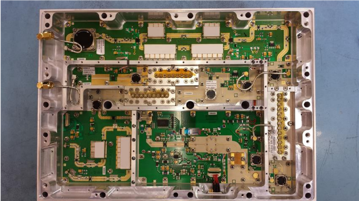
DTX-A213 LNA
