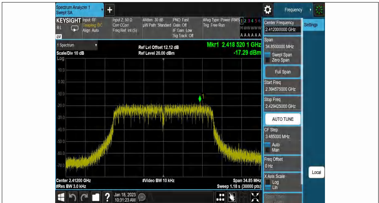
11N20SISO-Ant1-2412--17.30-0.00-0.00-0.00
