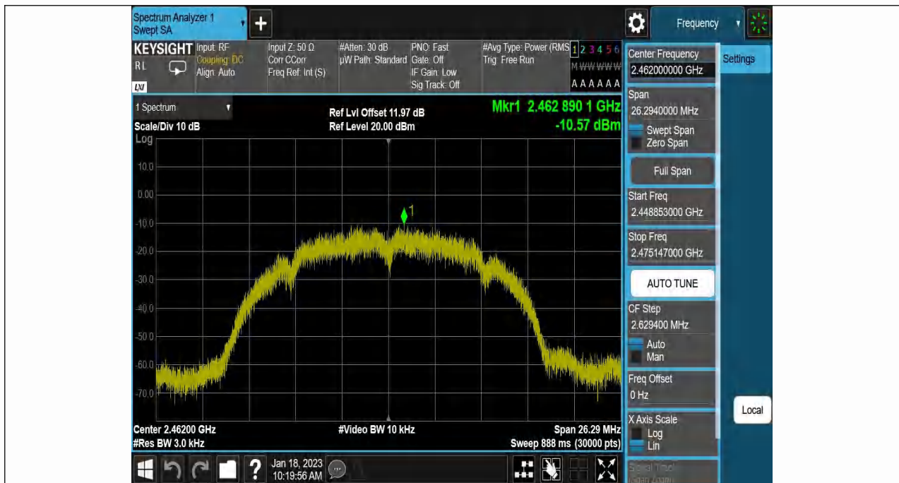
11B-Ant1-2462--10.57-0.00-0.00-0.00
