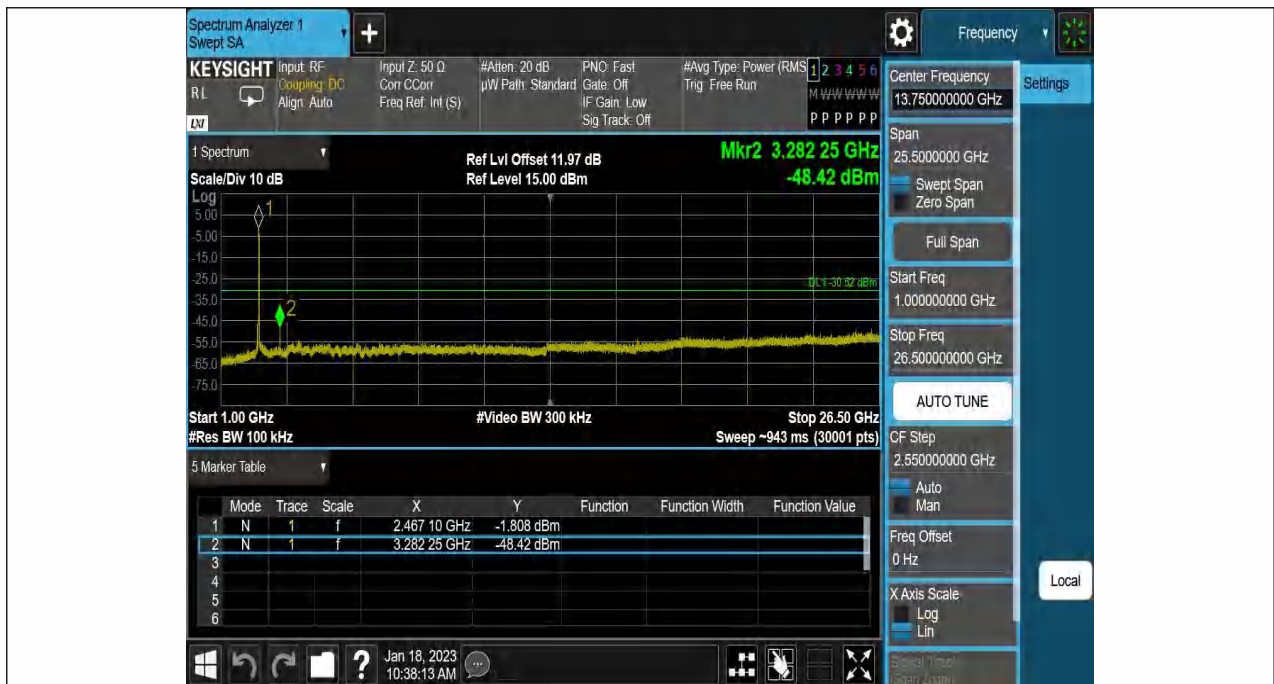
11N20SISO-Ant1-2462-1000~26500--0.52
