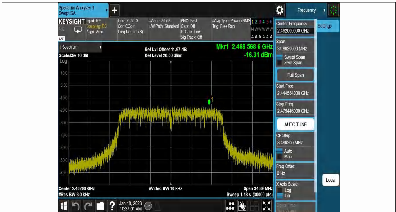
11N20SISO-Ant1-2462--16.31-0.00-0.00-0.00
