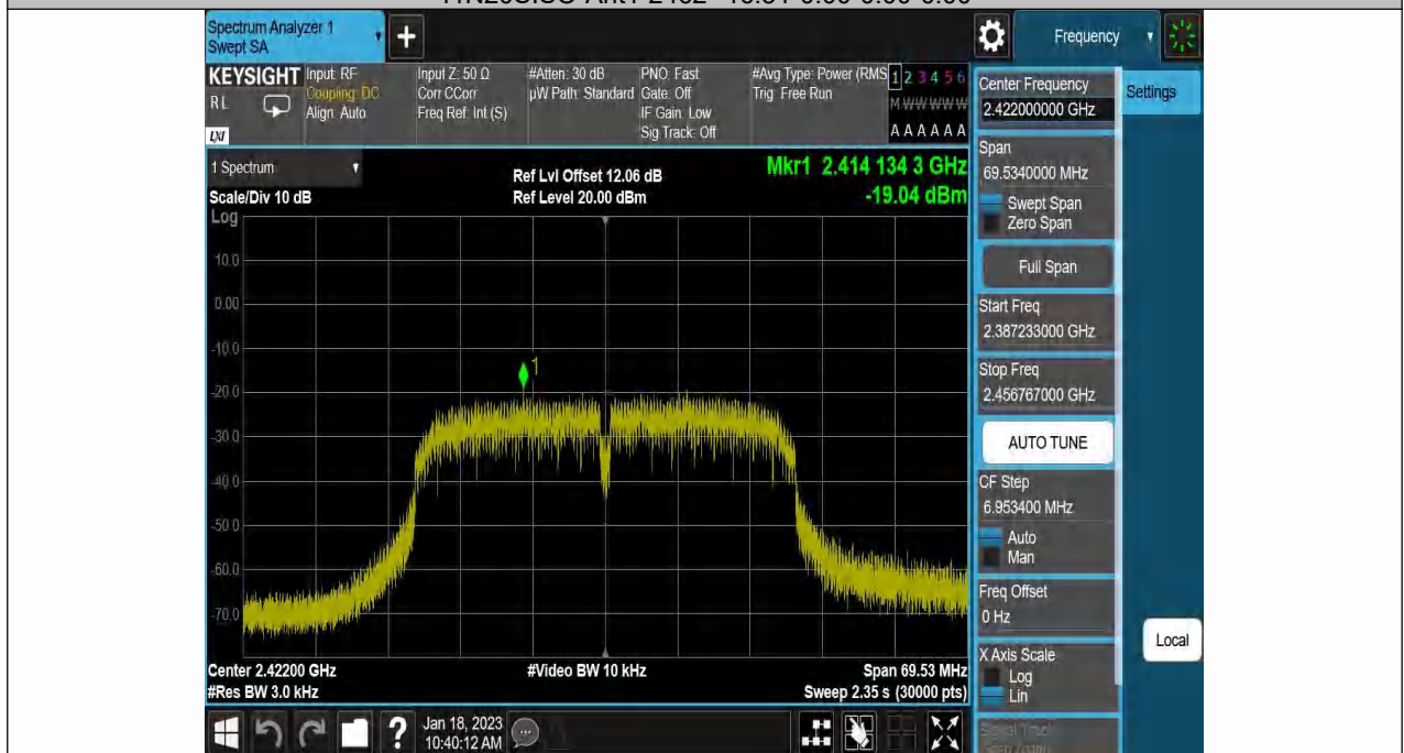
11N40SISO-Ant1-2422--19.04-0.00-0.00-0.00
