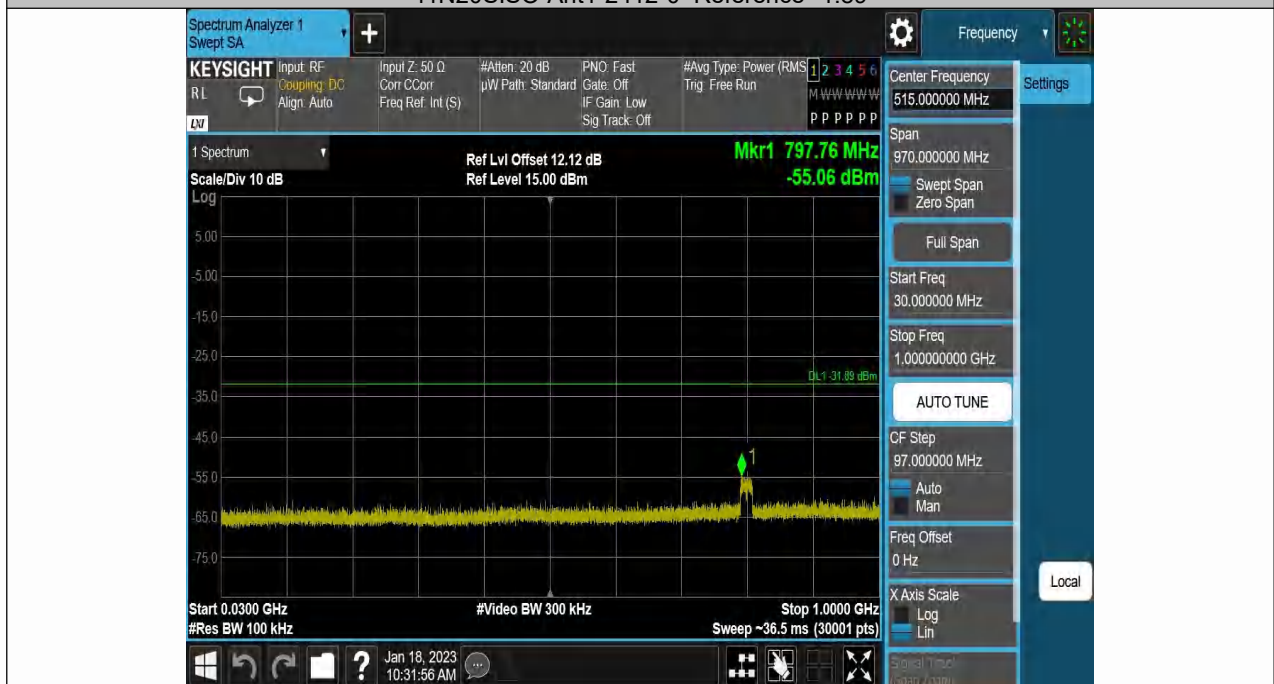
11N20SISO-Ant1-2412-30~1000--1.89
