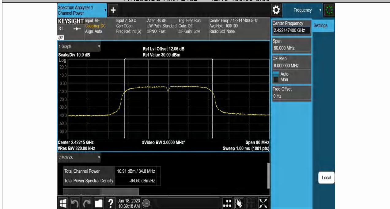
11N40SISO-Ant1-2422-----10.91-100.00-0.00
