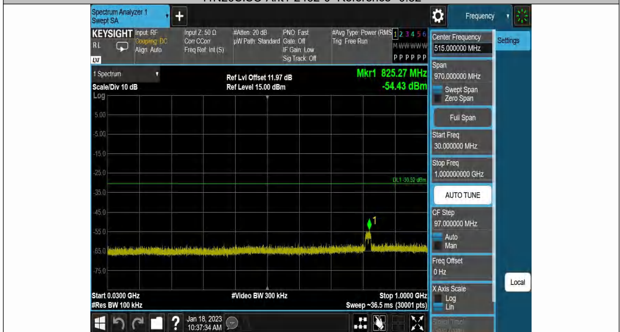
11N20SISO-Ant1-2462-30~1000--0.52
