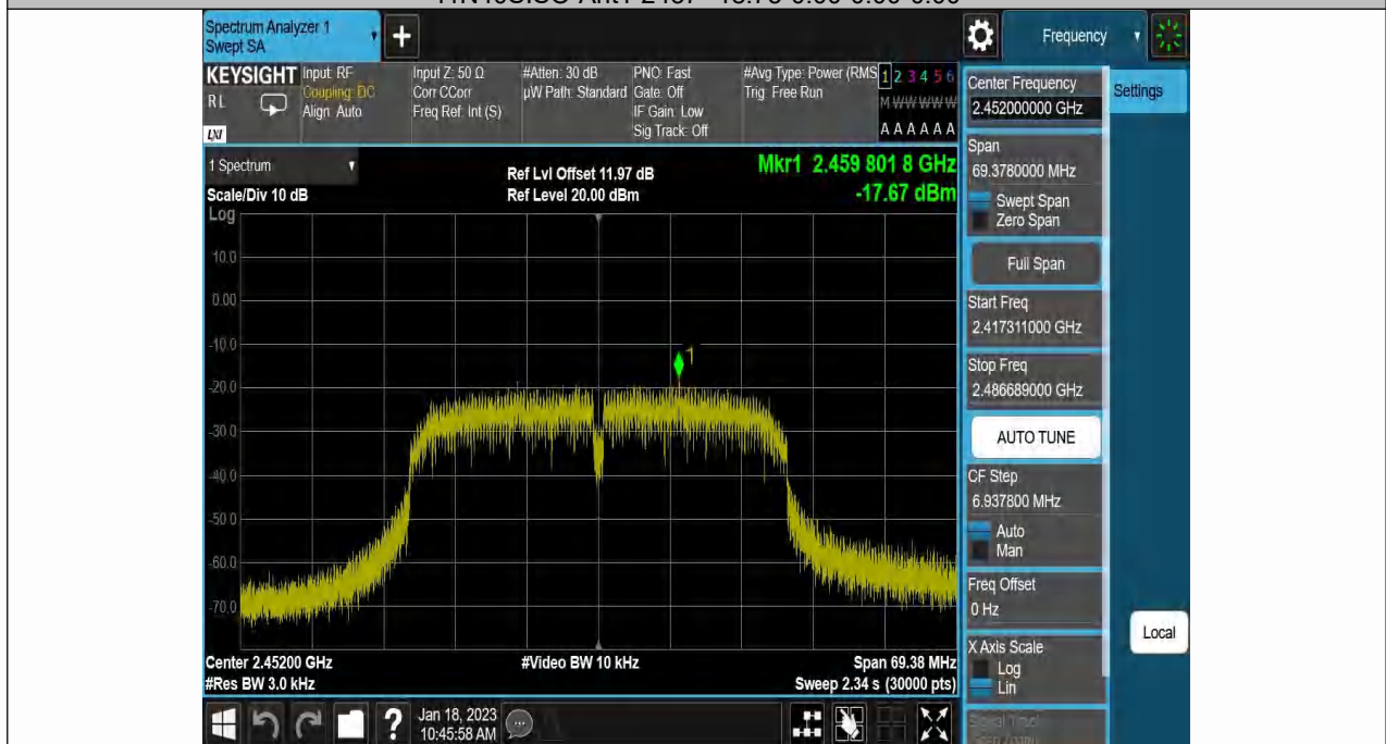
11N40SISO-Ant1-2452--17.67-0.00-0.00-0.00
