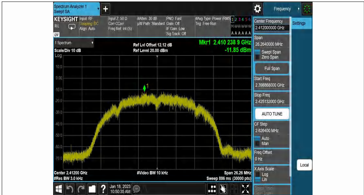
11B-Ant1-2412--11.85-0.00-0.00-0.00
