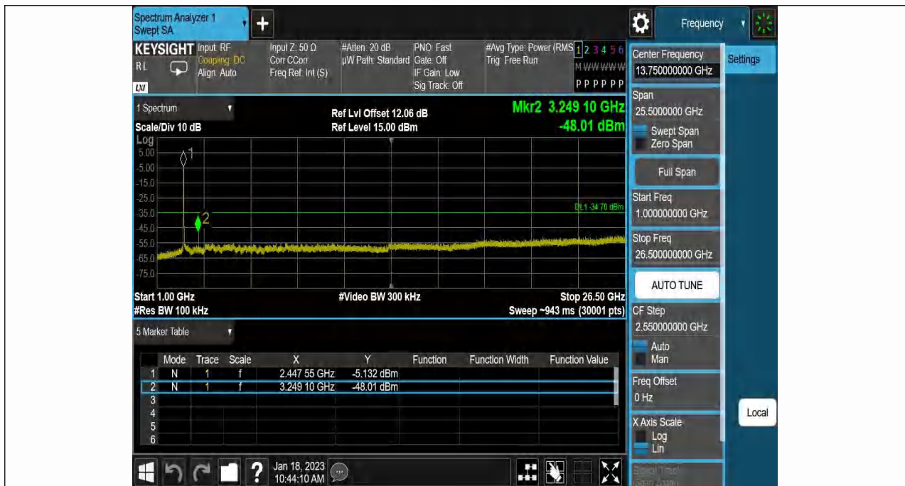
11N40SISO-Ant1-2437-1000~26500--4.70
