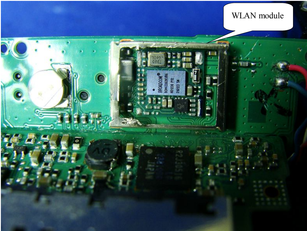
(22) EUT Photo (WLAN Module)
