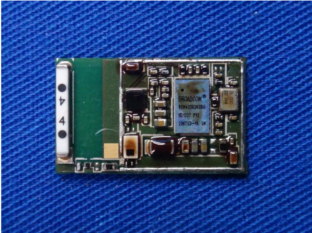
(21) EUT Photo
