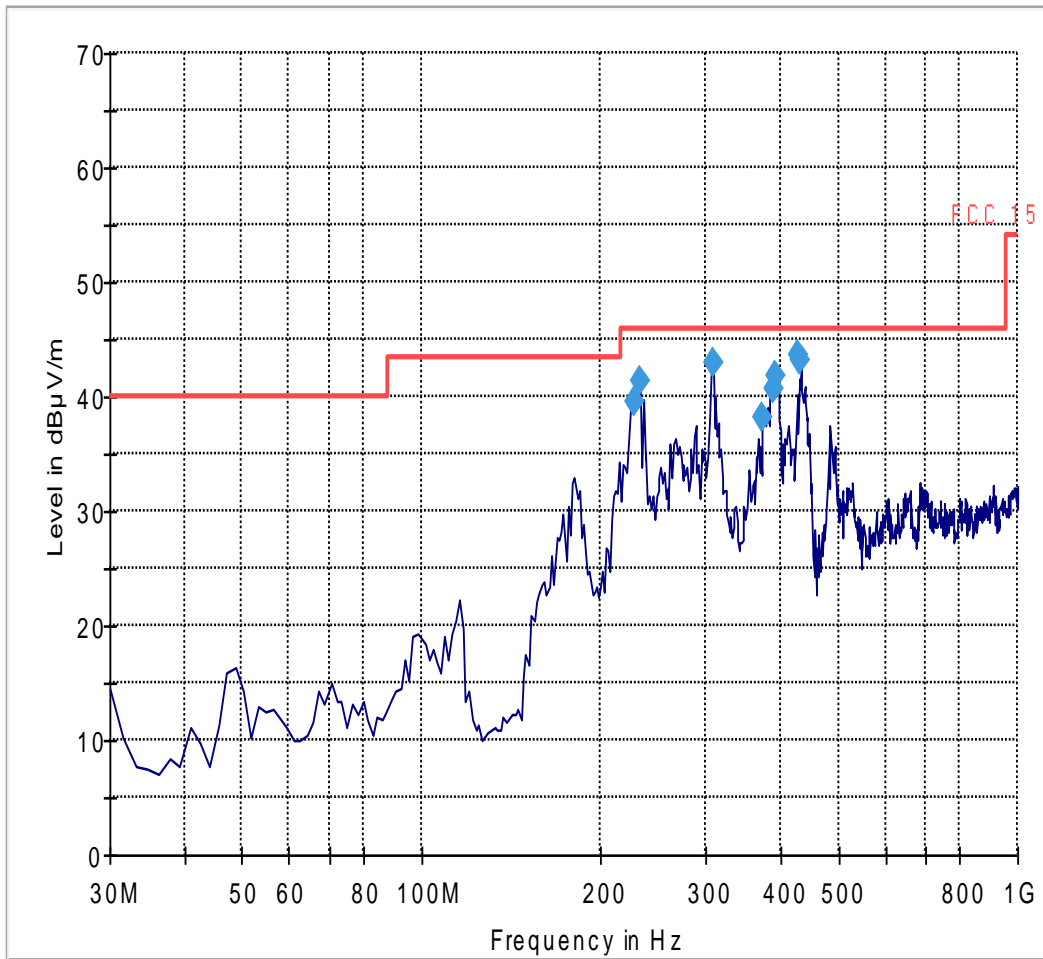
FCC 15 30-1000MHz
