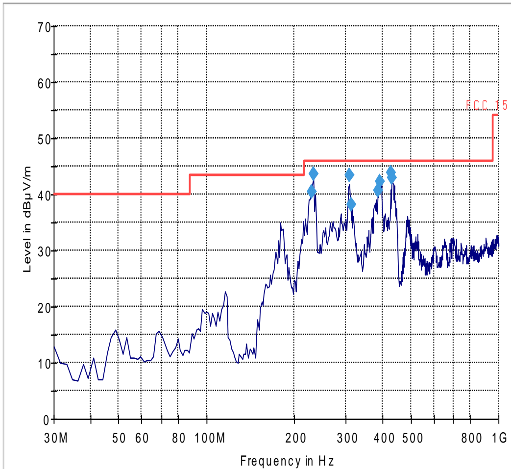
FCC 15 30-1000MHz
