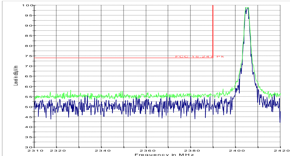
FCC 15.247 LBE Pk 3m
