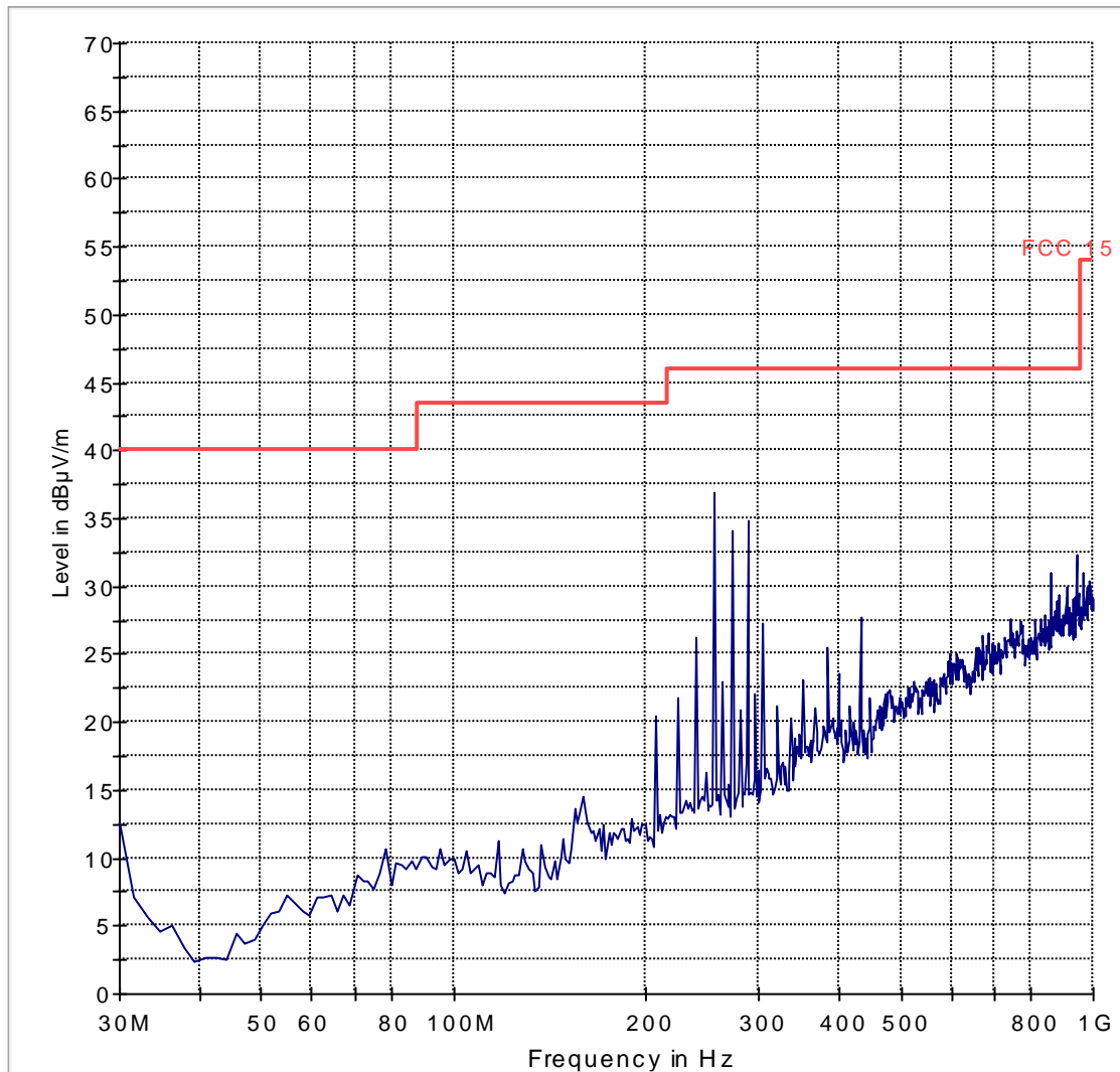
FCC 15 30-1000MHz
