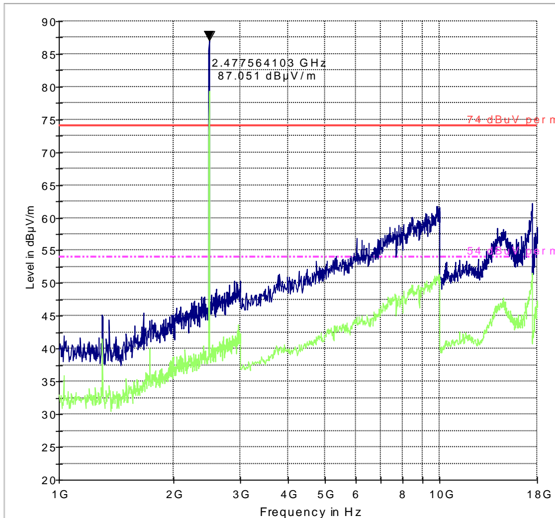
FCC 15 1-18GHz
