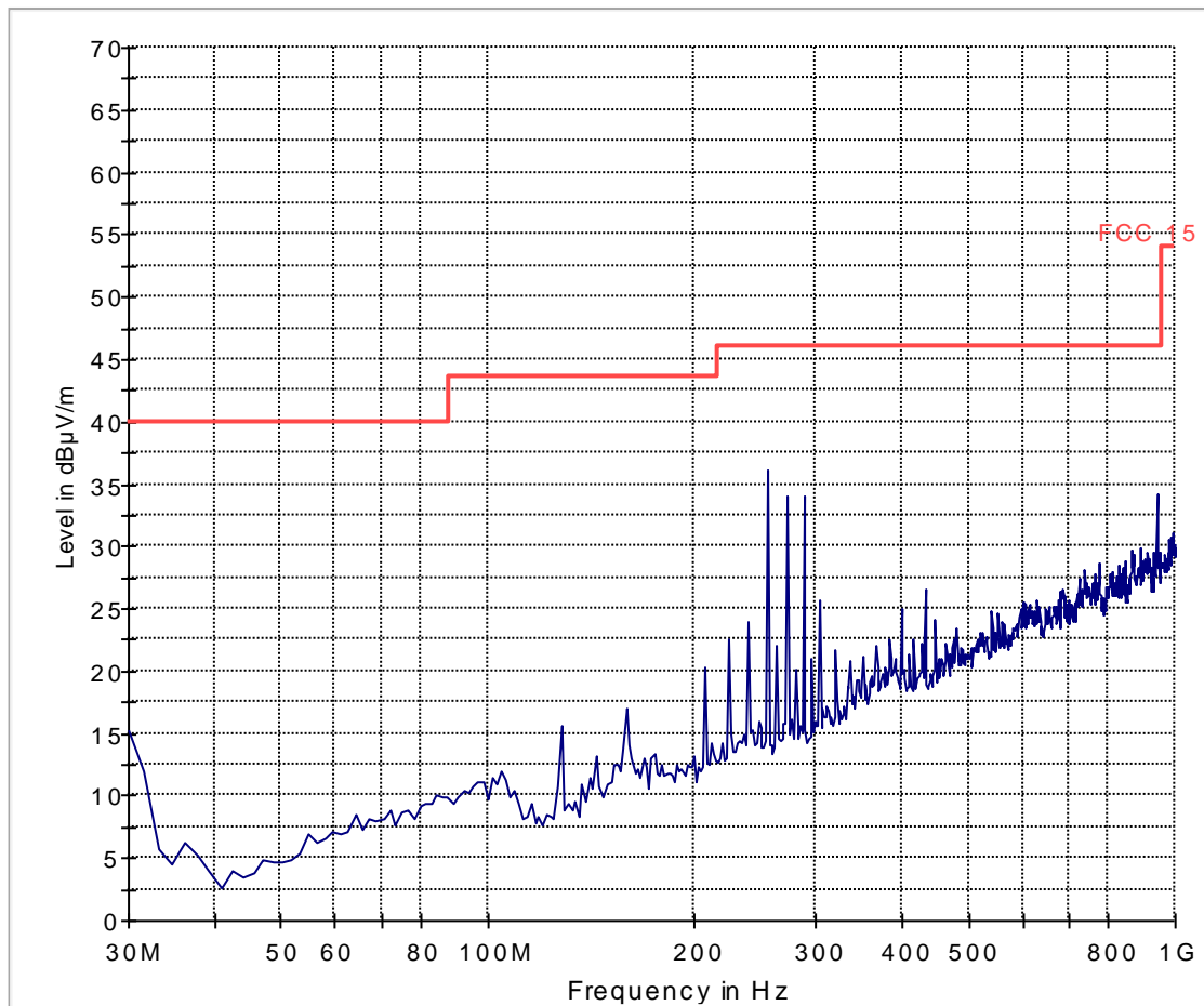
FCC 15 30-1000MHz
