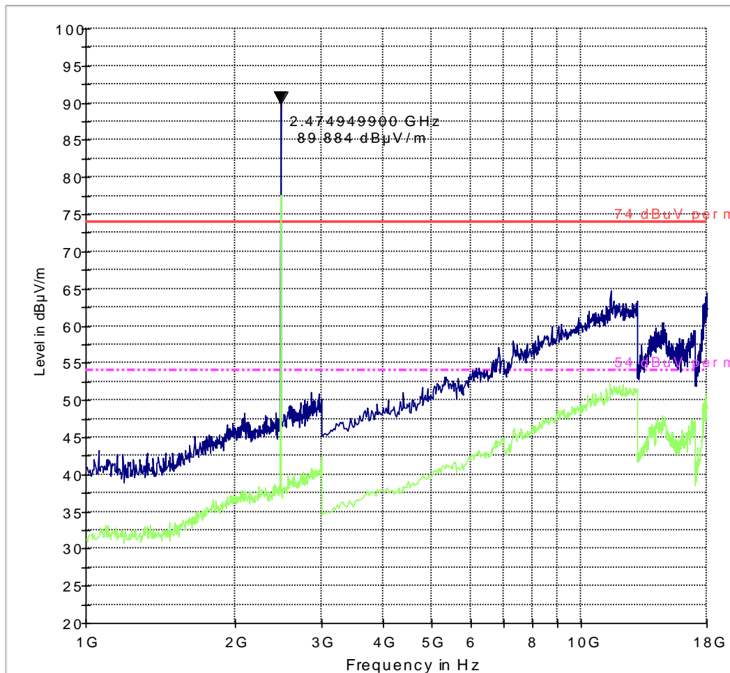
FCC 15 1-18GHz
