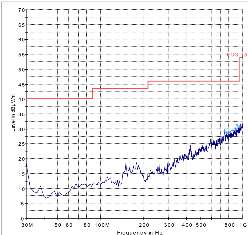
FCC 15 30-1000MHz
