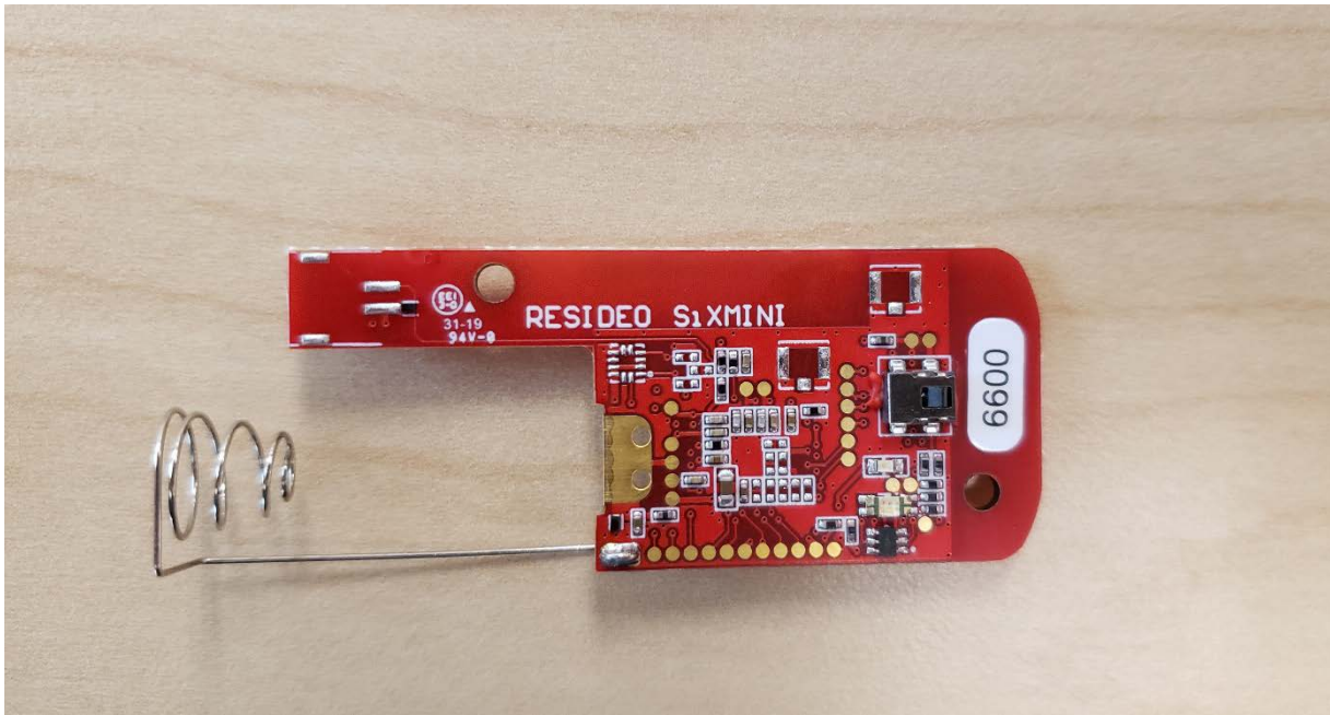
PCB Top
