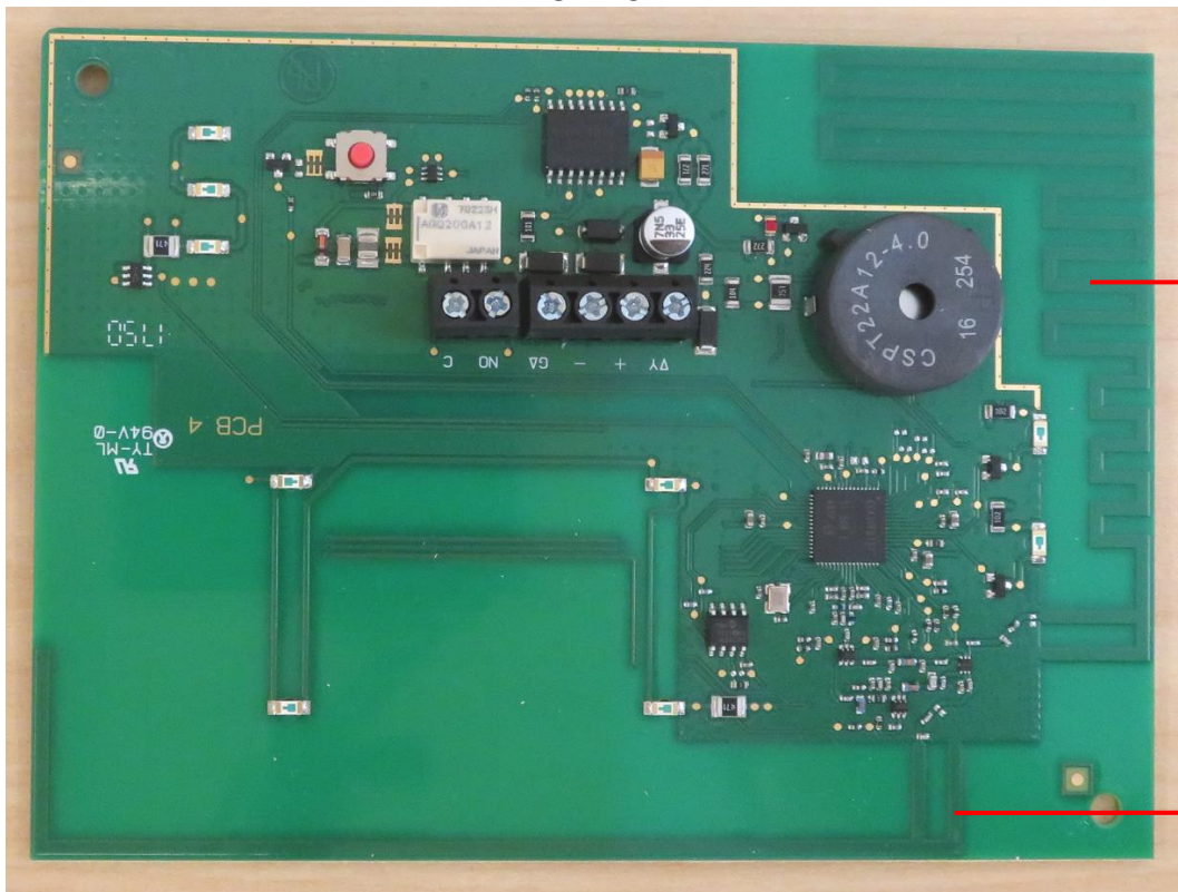
PCB TOP
