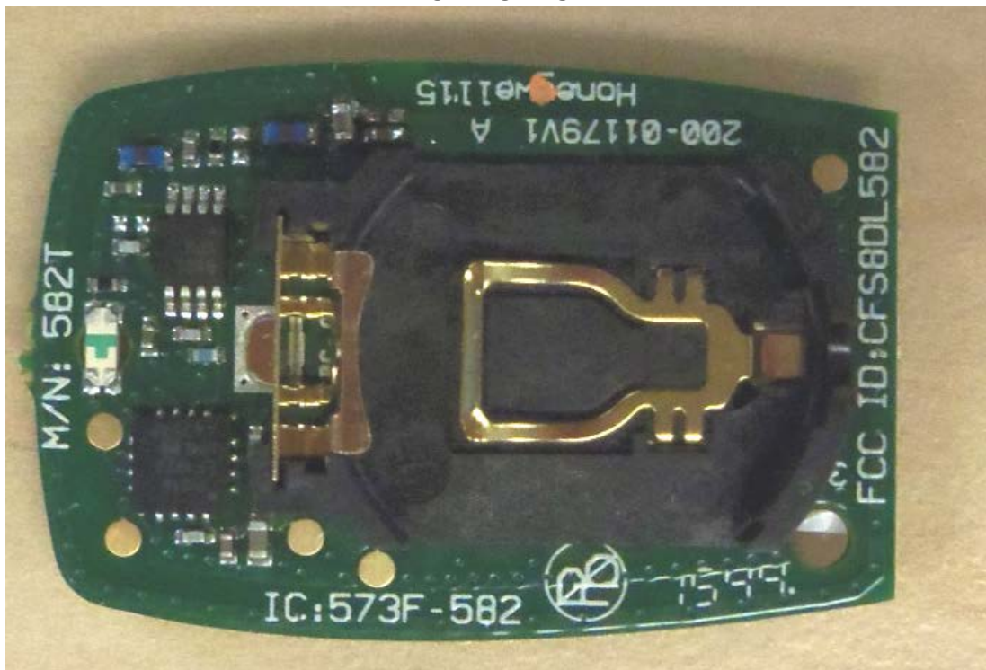
PCB BOTTOM
