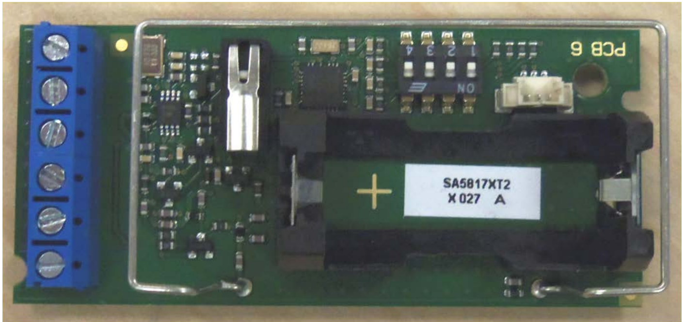
PCA TOP:
