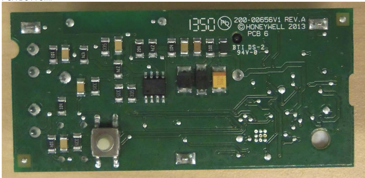
PCA BOTTOM:
