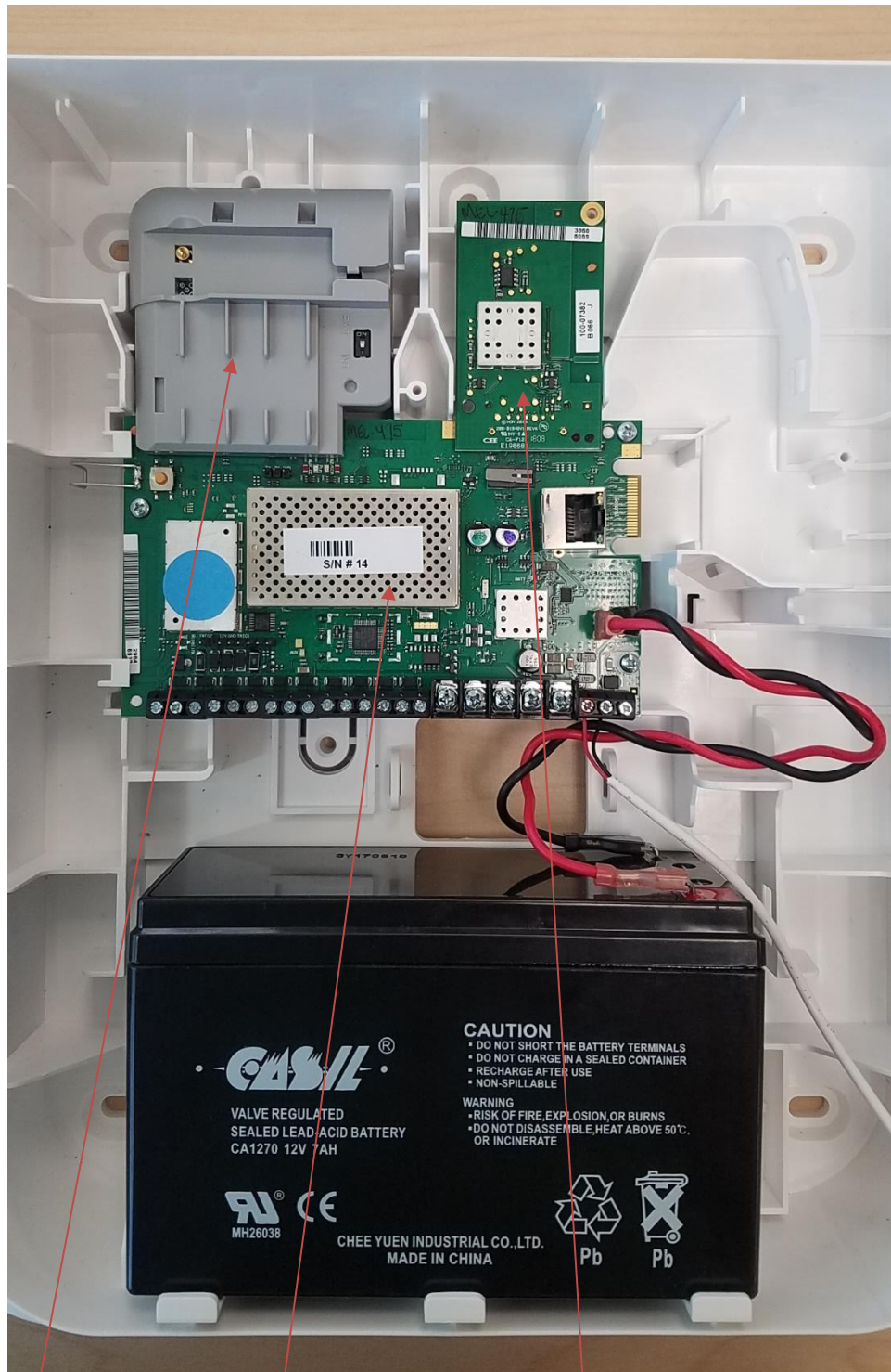
Cellular Module
