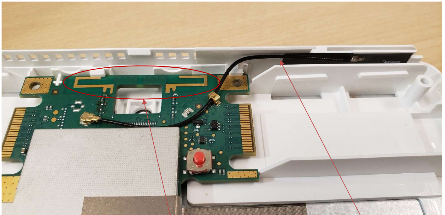
RF6 – Antenna 1 / BLE Antenna
